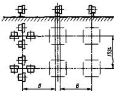
Трансформаторы массой 200-255 т
