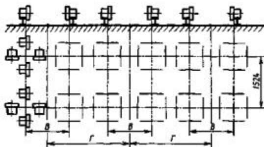
Трансформаторы массой 300-700 т
